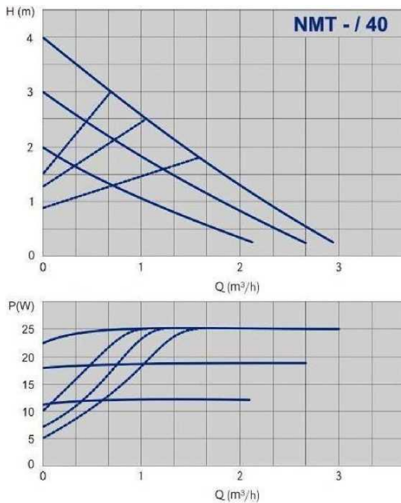
Рисунок 11 - Характеристики насоса
